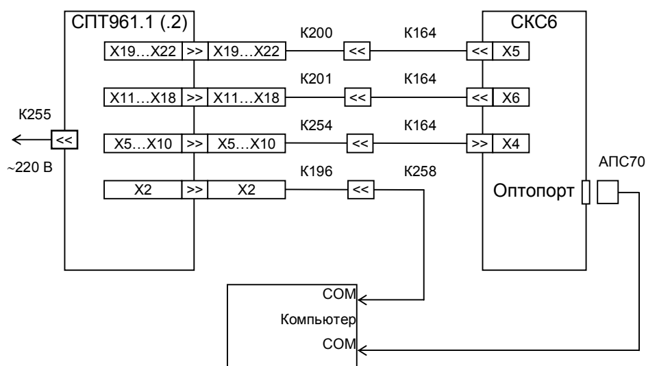
Рисунок 9.1 Схема проверки
