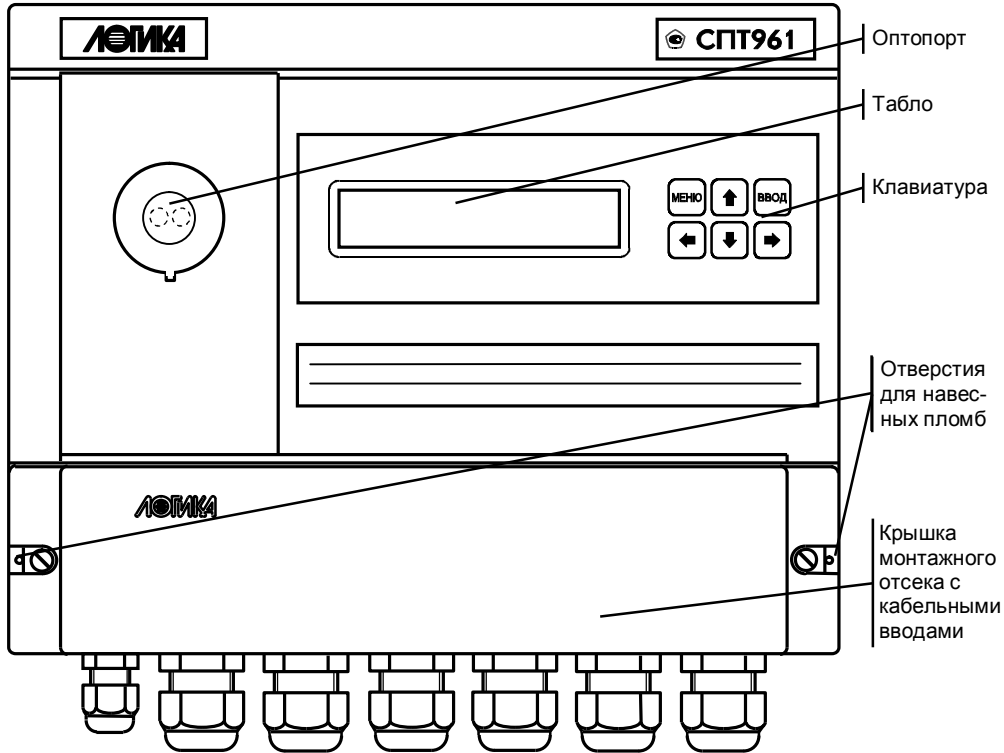
Рисунок 3.1 – Вид спереди
