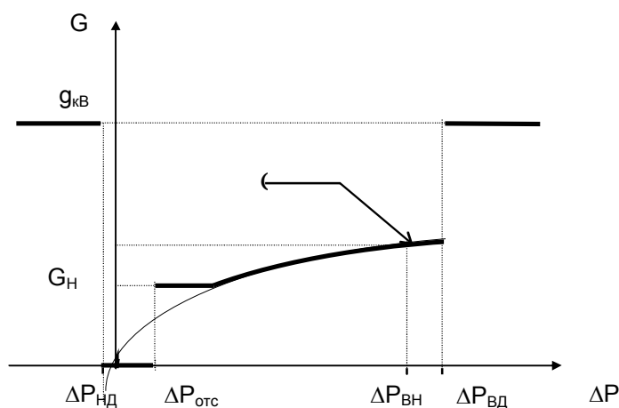
Рисунок 2.9 – Вычисление массового расхода по значениям перепада давления
