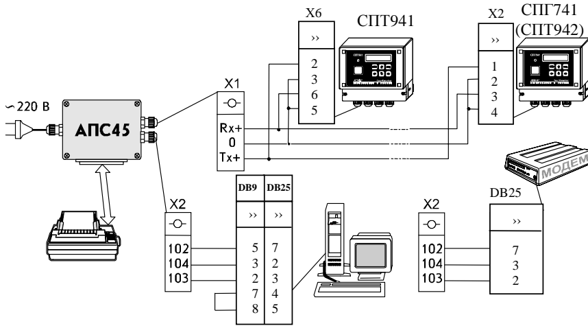
Рисунок 1 Схема подключения адаптера
