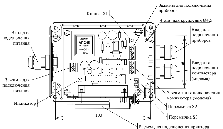
Рисунок 2 Конструкция адаптера. Крышка снята
